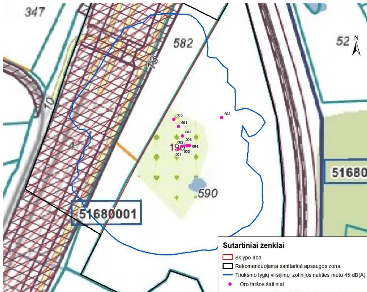
14 pav. SAZ riba su pažymėta nakties triukšmo izolinija
