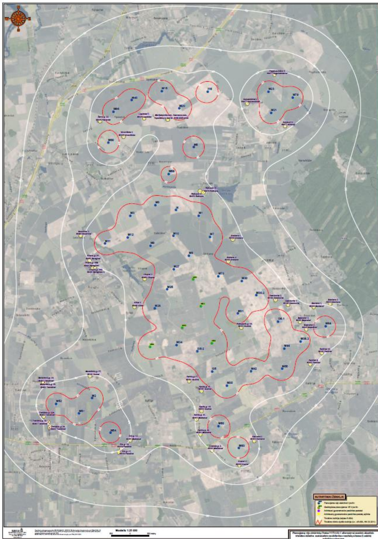
3 pav. Planuojamų vėjo elektrinių (Vestas V172 6.8, C alternatyva) suminio akustinio triukšmo sklaidos matematinio modeliavimo rezultatų schema (Lnaktis) pritaikius priemones
