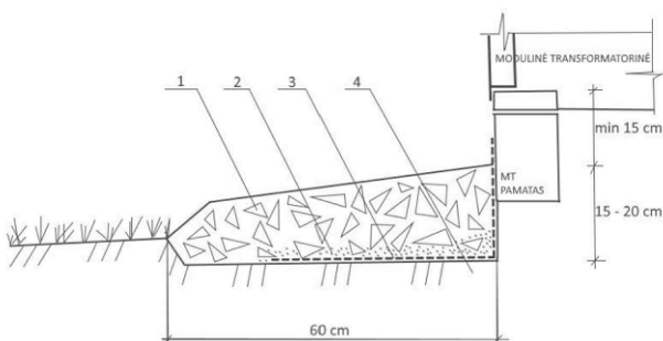
Detalè "A"
