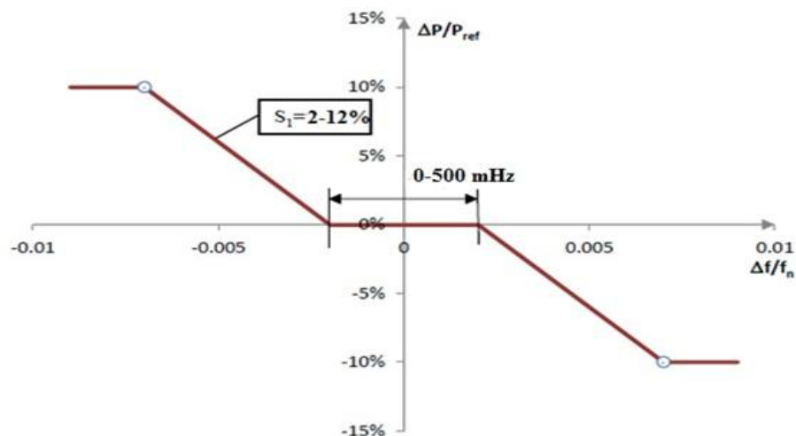
Pav. Nr. 2 Aktyviosios galios atsako į dažnio pokytį parametrai
