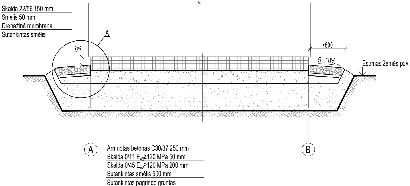
MT montavimo principinis vaizdas
