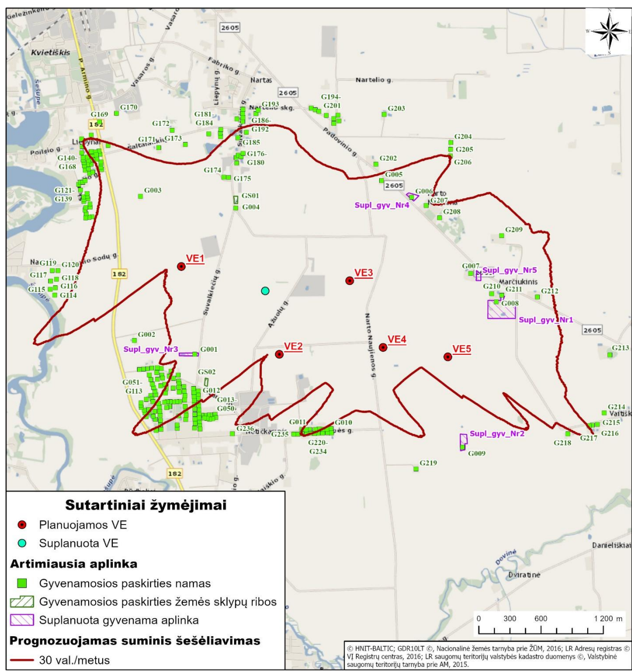
2 pav. Prognozuojamos suminio sukeltamo šešėliavimo (blogiausio scenarijaus) izolinijų grafinis atvaizdavimas
