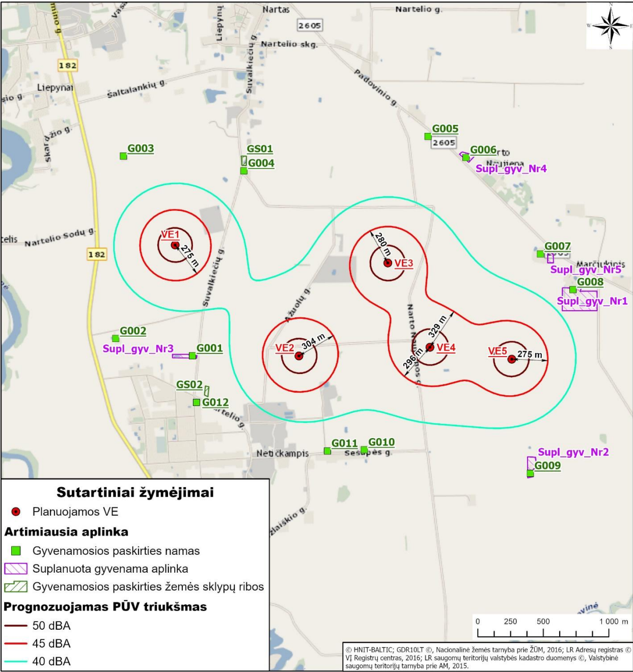
1 pav. Prognozuojamo PŪV triukšmo lygio izolinijos
