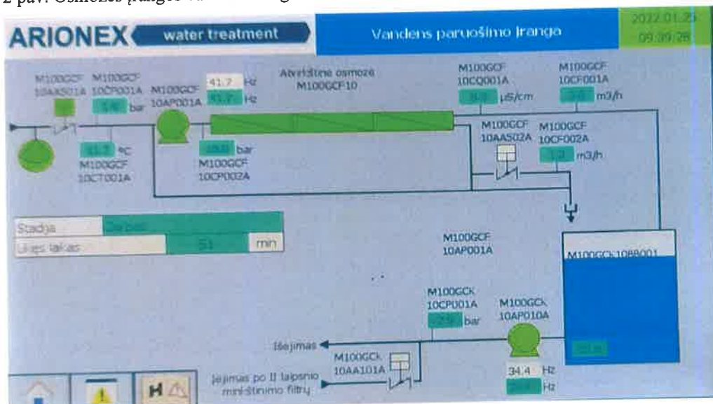
2 pav. Osmozės įrangos valdiklio langas
