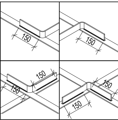
Įžeminimo sistemos stačiakampių profilių jungiamųjų laidininkų suvirinimo elektrolankinių būdų pavyzdys
