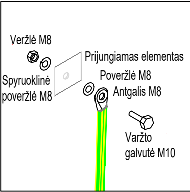
Įžeminimo laido tvirtinimas
