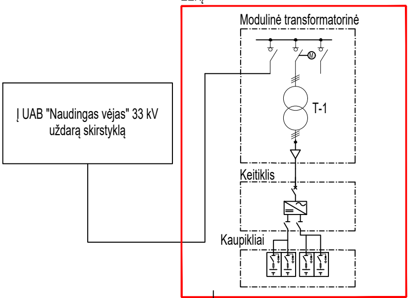
Principinė elektros energijos kaupimo įrenginio (EEK) prijungimo schema
