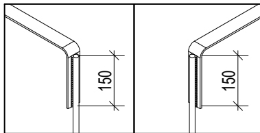
Įžeminimo sistemos apvalaus ir stačiakampių profilių jungiamųjų laidininkų suvirinimo elektrolankinių būdu pavyzdys
