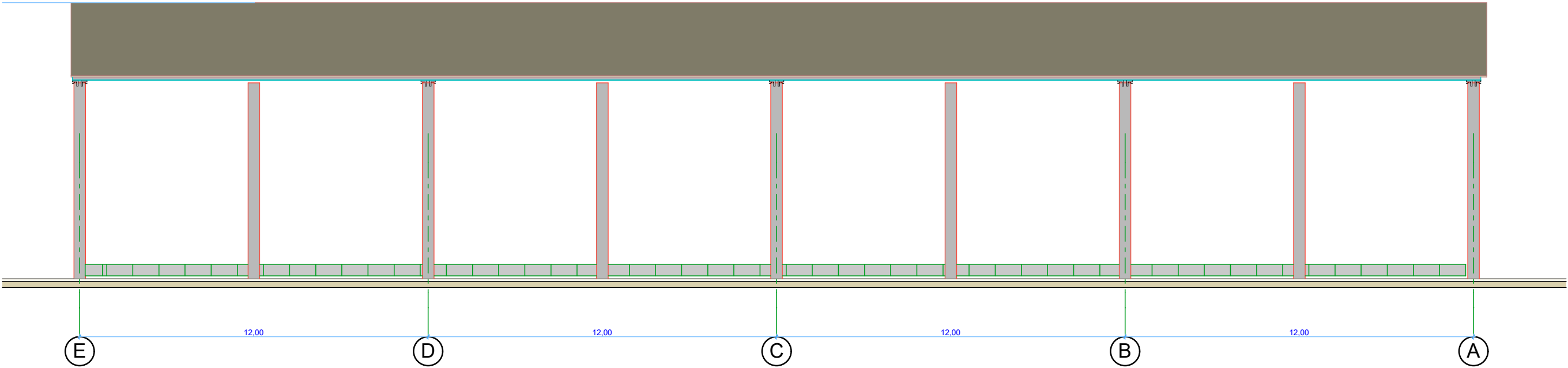
3 Fasadas E-A 1:150
