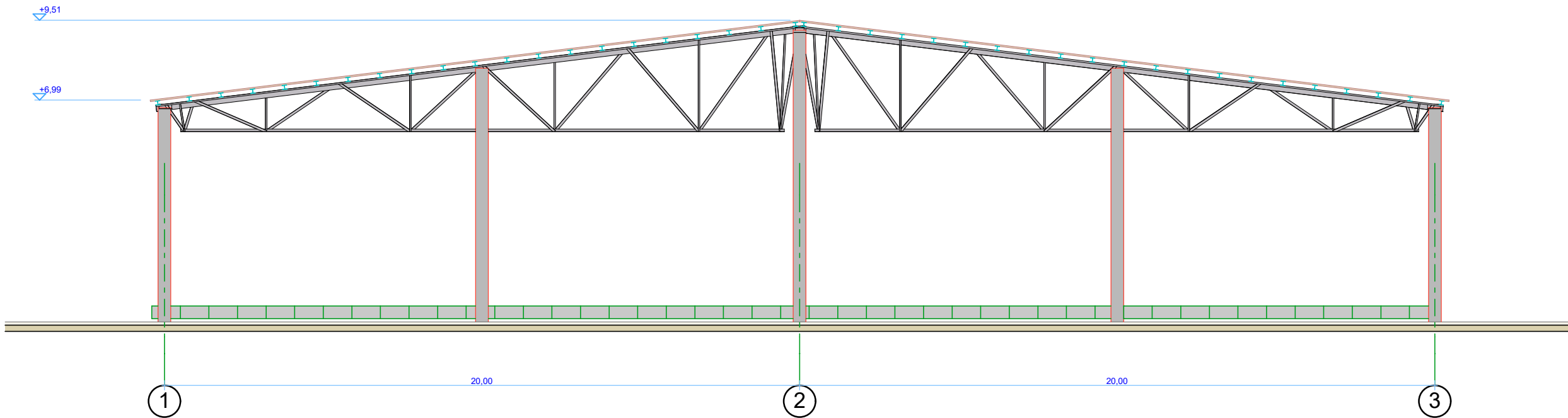
3 Fasadas 1-3 1:150
