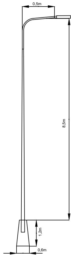
ŠVIESTUVO ESKIZAS
